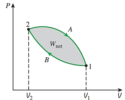
Fig.1.11 - Cycle
